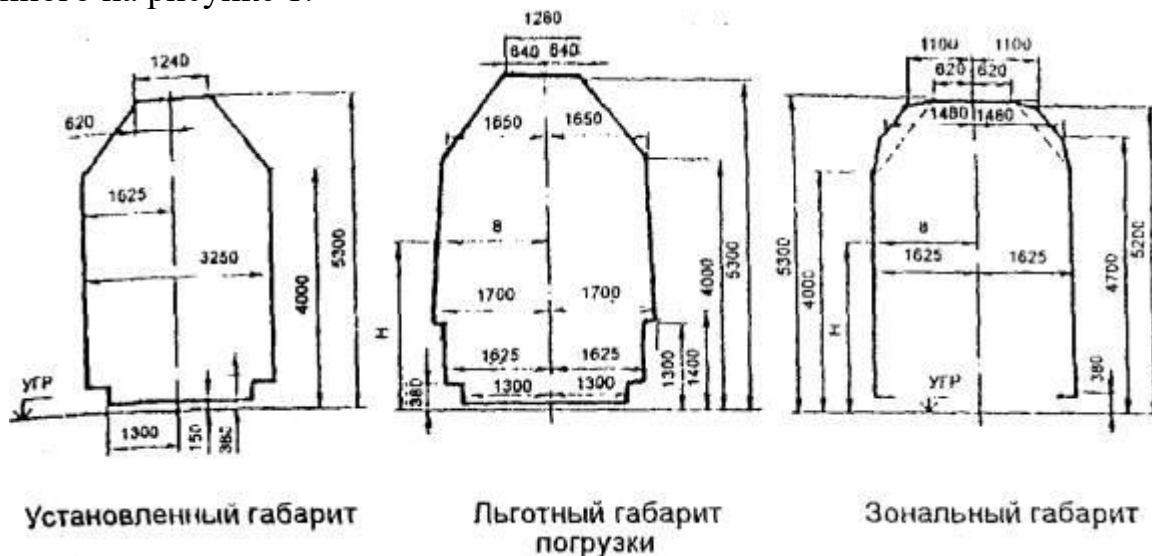
Рисунок 1 - Габариты погрузки грузов в железнодорожные вагоны
